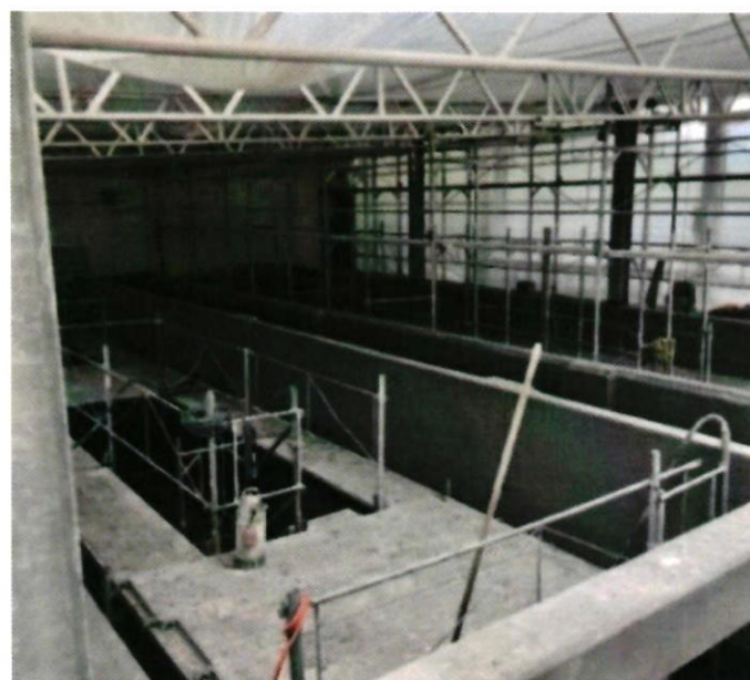
Bild: Becken während der Beschichtungsphase
