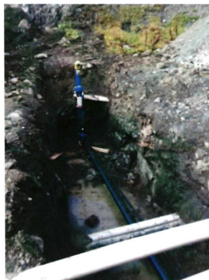
Bild: Versetzung bestehender Hydrant wegen Neubau Carmennahütte
