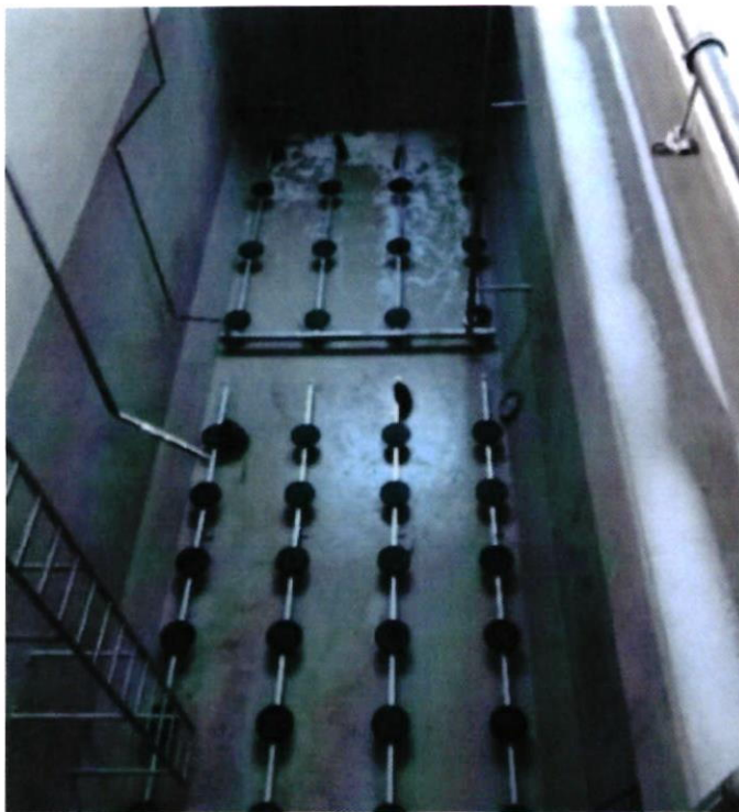
Bild: Montage der neuen Belüftungsteller
