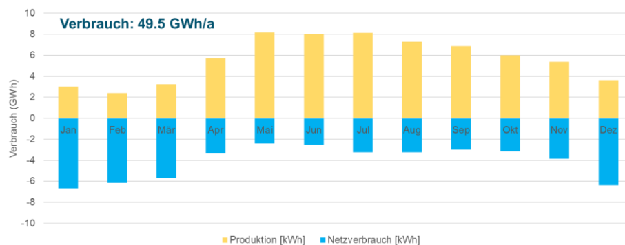
Abbildung 9: Übersicht Verbrauch und Erzeugung im Gemeindegebiet Arosa
