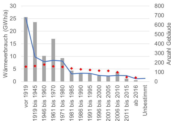
Abbildung 13: Gebäudebestand in Arosa aufgeschlüsselt nach Alter der Gebäude (blau) jeweiliger Energiekennzahl (EKZ in rot) und Wärmeverbrauch (graue Balken).
