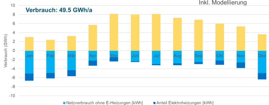
Abbildung 10: Darstellung des Stromverbrauchsanteil der Elektroheizungen inkl. Modellierung (ca. 14 % an totalem Stromverbrauch)
