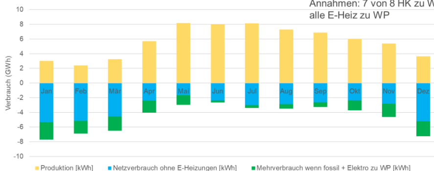
Abbildung 12: Ersatz der fossilen Heizungen und Elektroheizungen mit Wärmepumpen.
