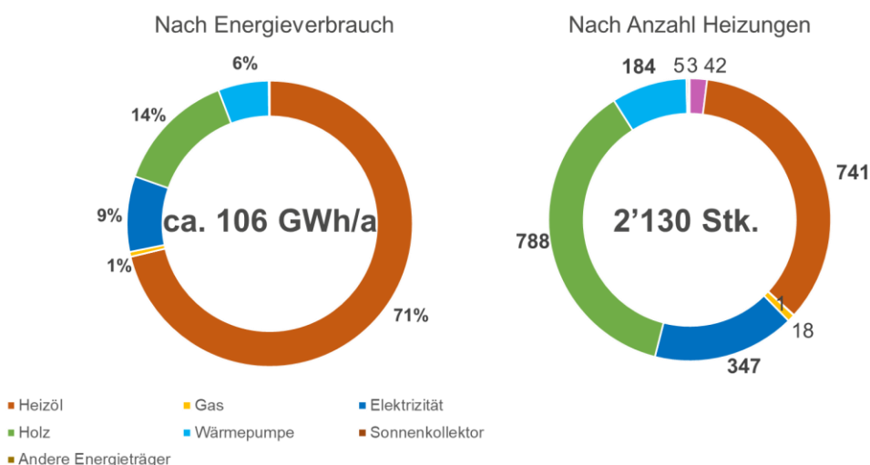
Abbildung 4: Wärmebedarf für Heizung und Warmwasser nach Energieverbrauch und Energieträger in der Gemeinde Arosa
