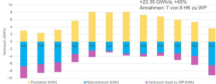
Abbildung 11: Ersatz der fossilen Heizungen ohne Elektroheizungsersatz.
