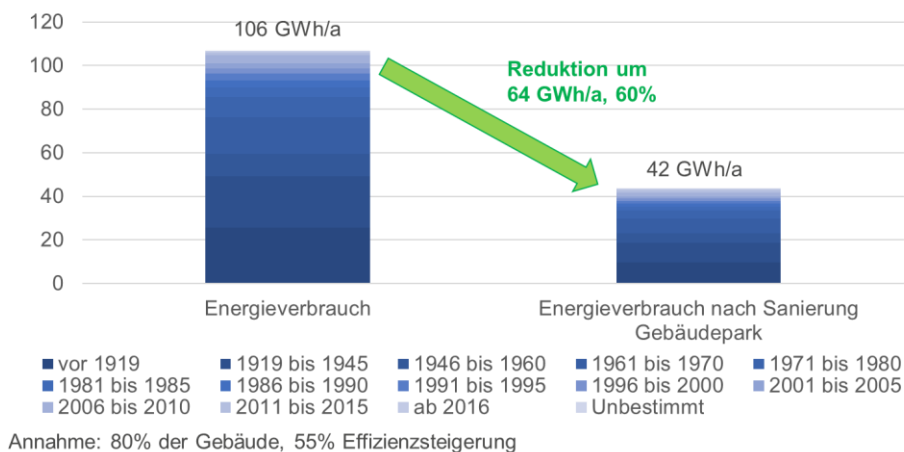
Abbildung 14: Mögliche Einsparung bei Umsetzung von Effizienzmassnahmen.
