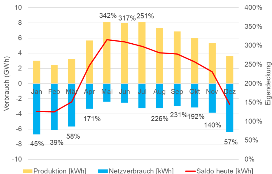
Abbildung 3: Jahresverbrauch und Produktion von Arosa Energie mit Deckungsgrad.
